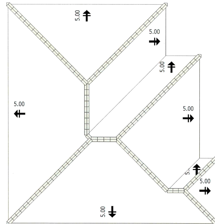
棟面積表
